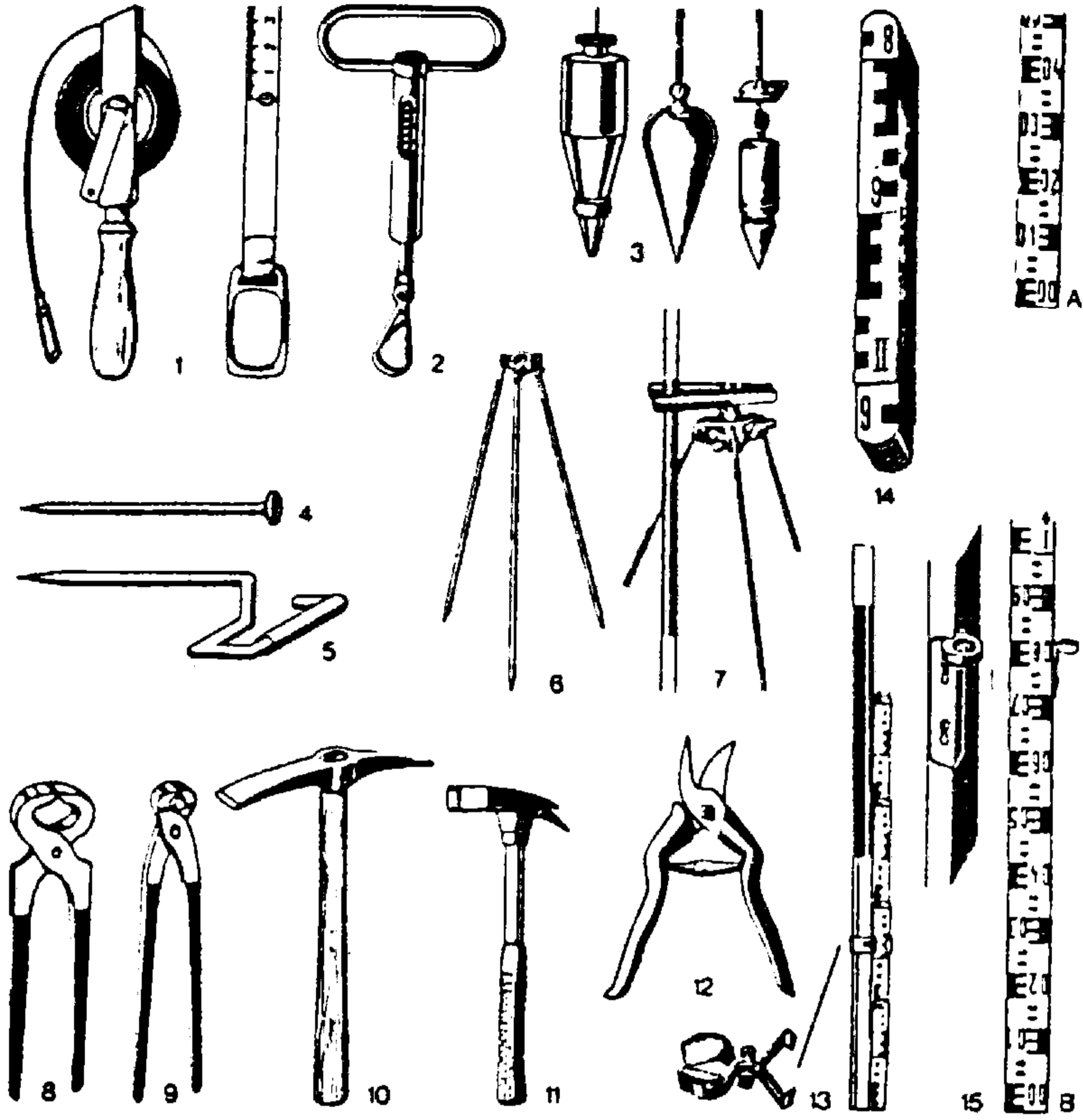
(شكل ٤) أدوات القياس في الحفائر
